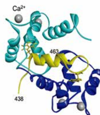
CaMKK(438-463)とCalmodulin複合体の立体構造解析 (PDB ID: 1cck)
