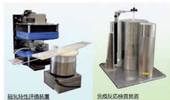
超高感度磁気計測システムの開発と免疫検査への応用
